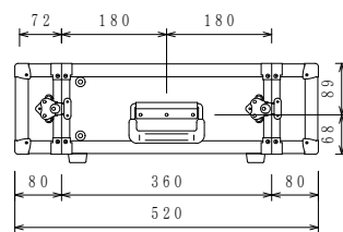
フタ内寸
